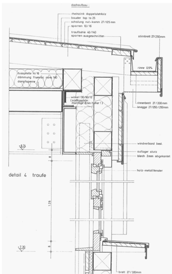
Detailschnitt Turnhallendach
